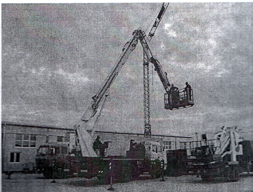
Slika 2. Hidraulična polužna kamionska dizalica sa platformom
